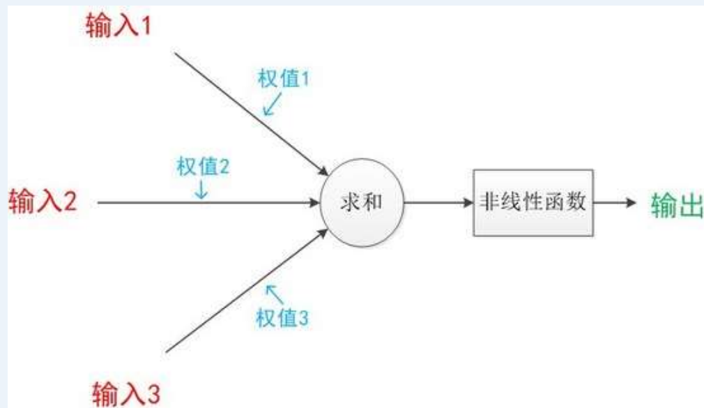
神经元模型
