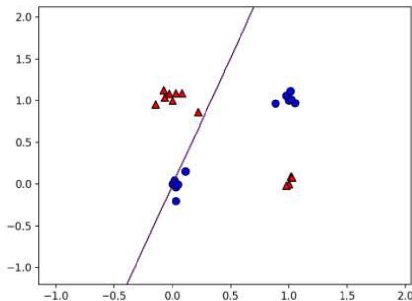
XOR任务
